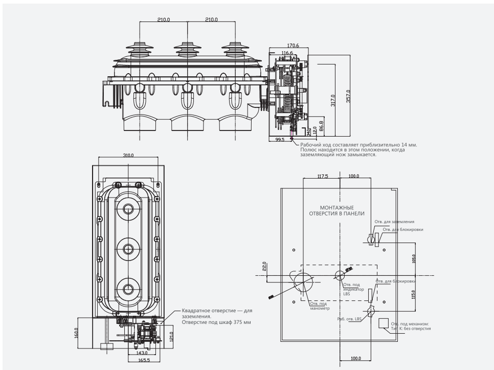
Рис. 2. Общая схема выключателя нагрузки
