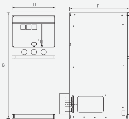
600×845×1550(Ш*Г*В) Ячейка подключения силового трансформатора без разъединителя (стандартный тип)
