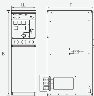
442×845×1550(Ш*Г*В) ячейка с выключателем нагрузки
