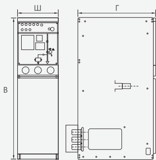
442×845×1550(Ш*Г*В) ячейка с выключателем
